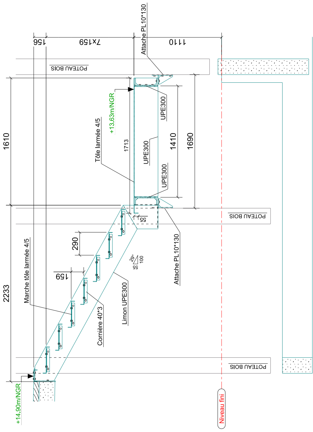
Coupe F - F 1:30
