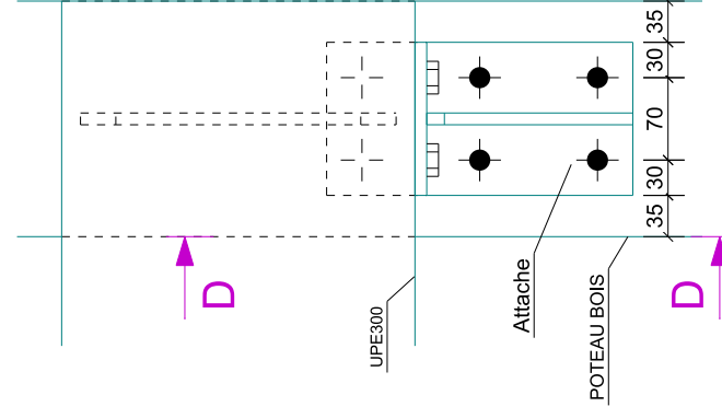
Détail F 1:7
