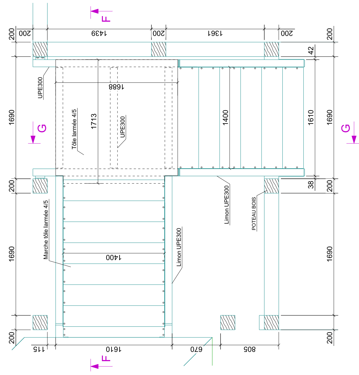
vue en plan 1:30
